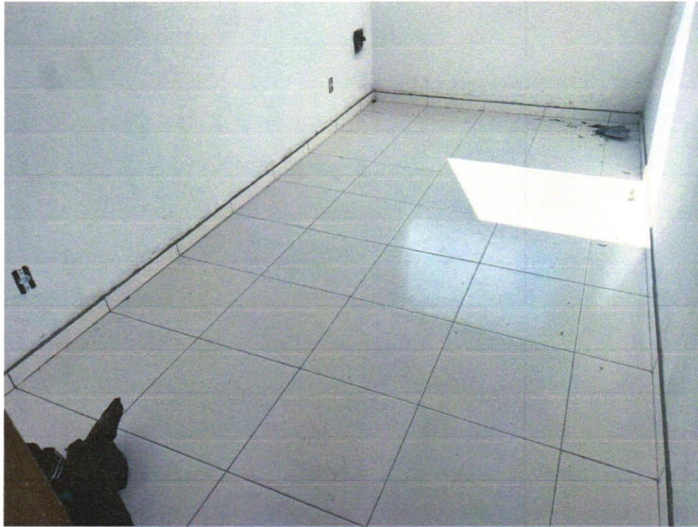
Foto 05- RODAPÉ CERÂMICO DE 7CM DE ALTURA COM PLACAS TIPO ESMALTADA EXTRA DE DIMENSÕES 45X45CM. AF_06/2014
